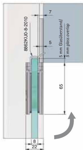
Türflügel einseitig 90° öffnend/ wing of the door opens in one direction 90°
