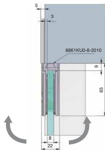
Türflügel beidseitig 90° öffnend/wing of the door opens in both direction 90°
