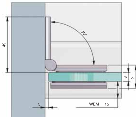
Türflügel einseitig 90° öffnend/ wing of the door opens in one direction 90°
