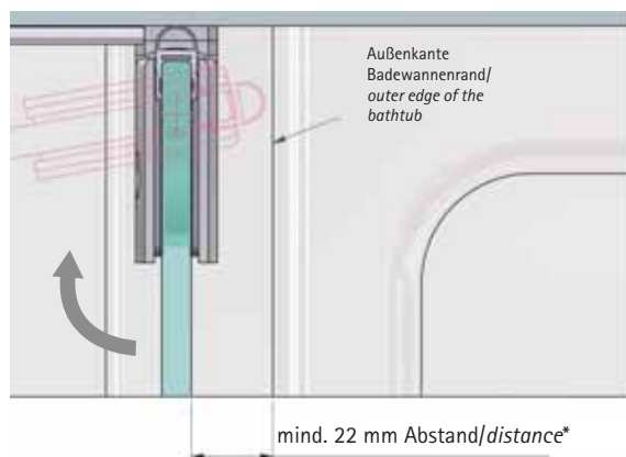
Türflügel einseitig 90° öffnend/wing of the door opens in one direction 90°
