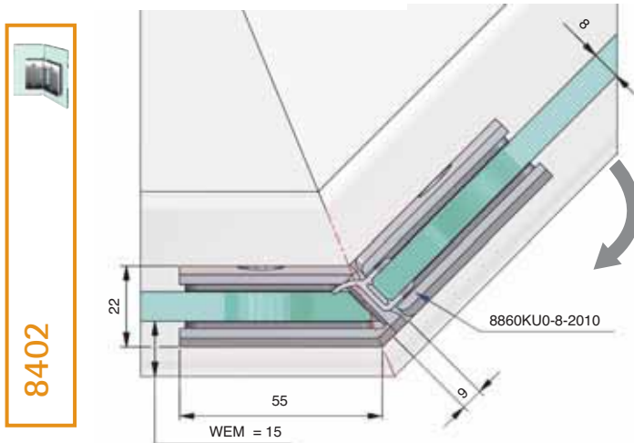
Türflügel einseitig 90° öffnend/ wing of the door opens in one direction 90°
