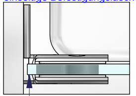
Duschtürband 8406MS einseitige Befestigungsglasche
