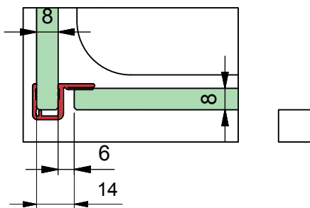
d) ohne Dichtprofil 8 mm Glas
