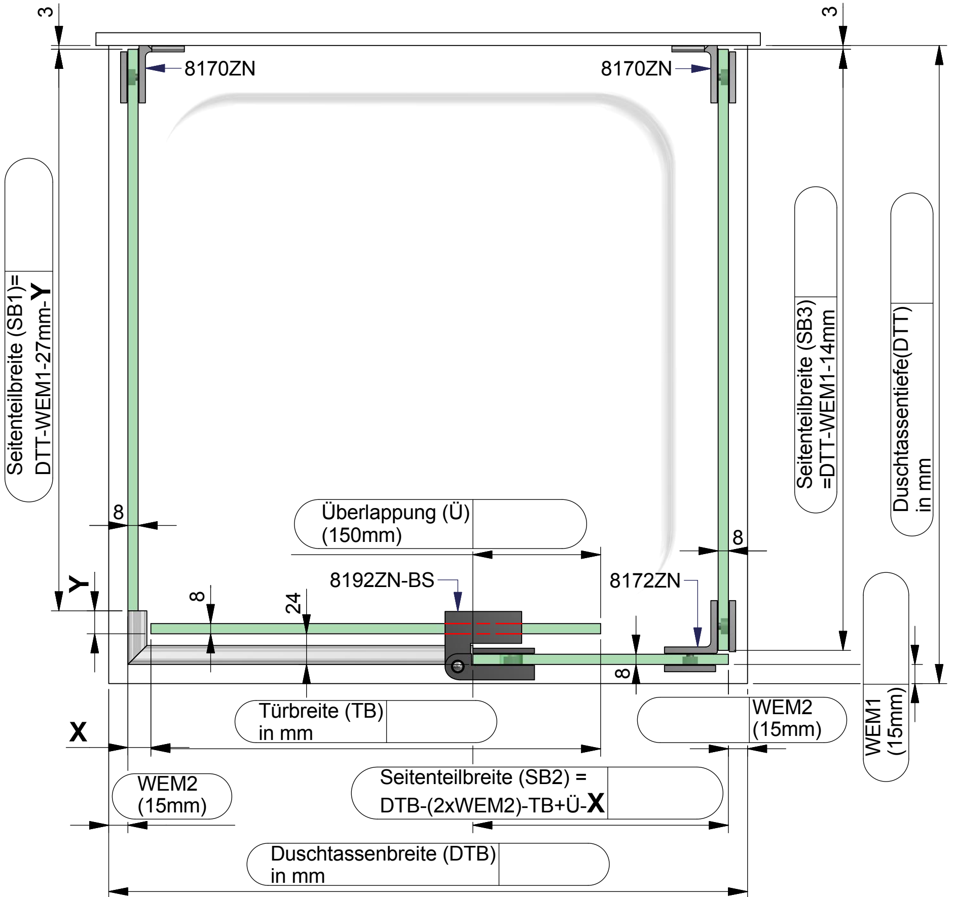
a) mit Dichtprofil 8851KU0-8
