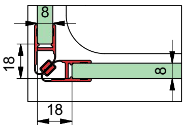
c) mit Dichtprofil 8861KU0-8
