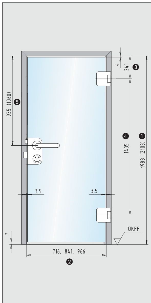
Glastürblatt mit Zarge - BBL = Mitte Band
