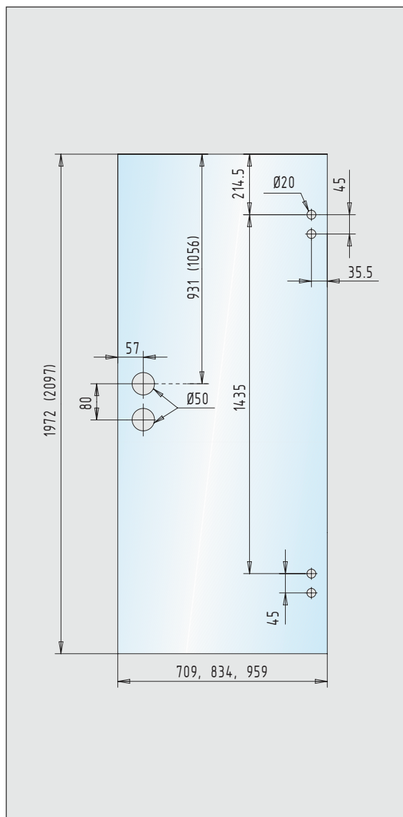
Glastürblatt für VX / VN / VS vorgerichtet
