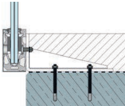
(B) Stirnseitiger Anschluss an Stahlunterkonstruktion mit Estrichabschluss
