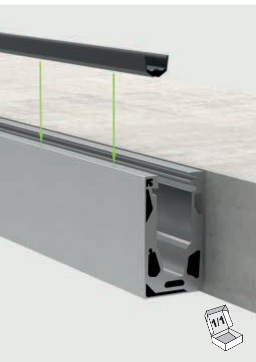
Verglasungsprofil | glazing profile
