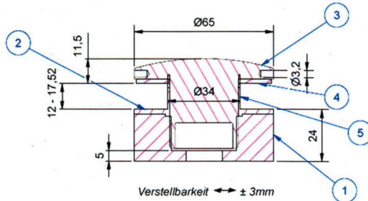
A-A (1 : 1,5)
