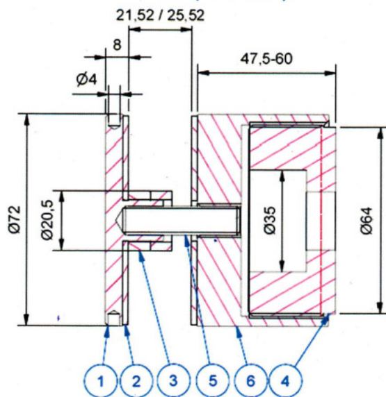
A-A (1:1,5)
