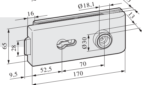
PZ-Schloss vorgerichtet für Profilzylinder
