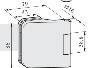
OBJEKT Türband mit Hülse für 24 mm Falztiefe (Objektbereich)
