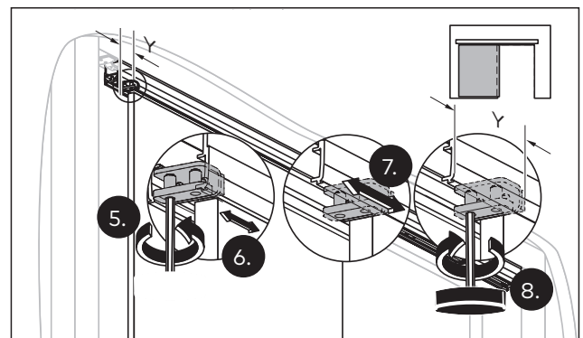
Abb. 40 Den Endanschlag in der Offen-Position positionieren
