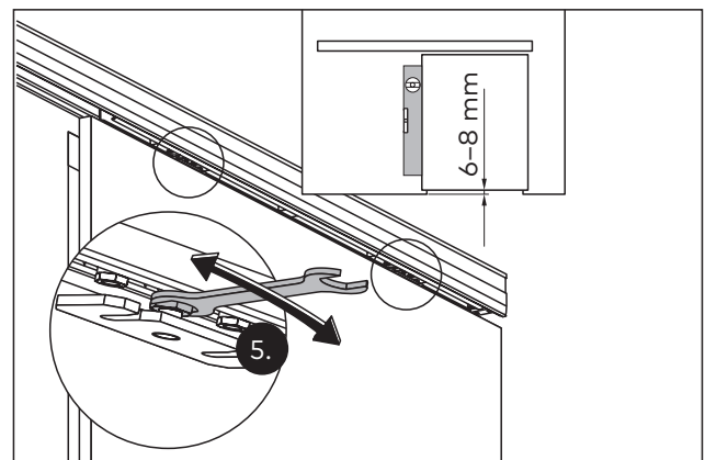
Abb. 20 Den Türflügel in der Höhe verstellen
