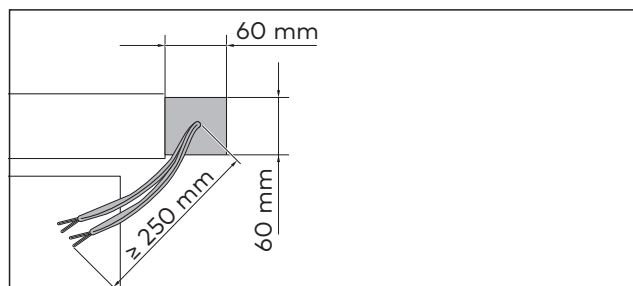
Abb. 5 Montage mit Festanschluss
