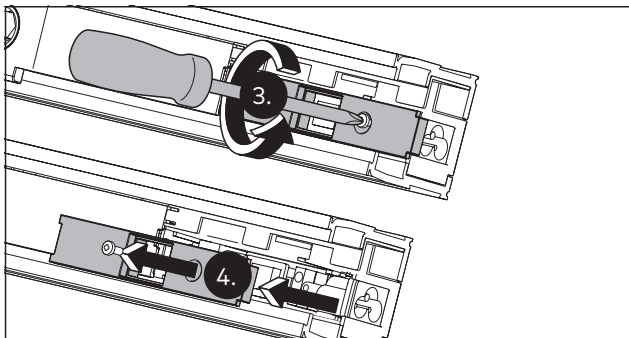
Abb. 41 Den Deckel entfernen
