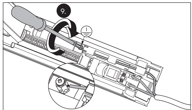
Abb. 45 Die Erdungsklemme anschließen
