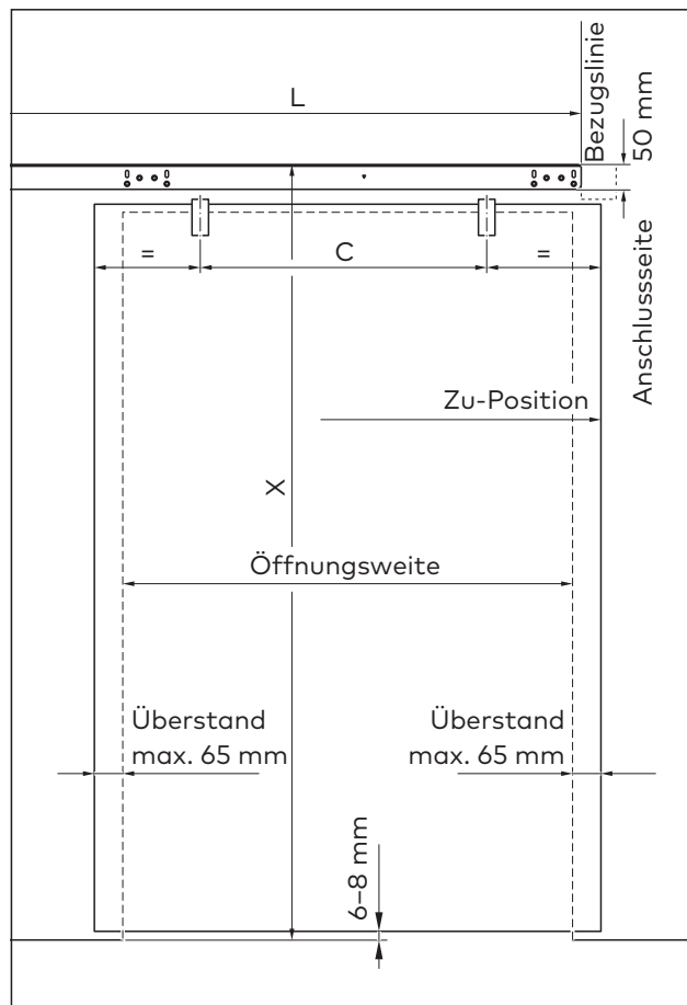
Abb. 9 Den Abstand X auf der Wand anzeichnen
