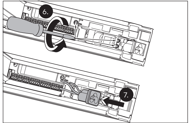
Abb. 43 Die Anschlussbuchse herausziehen
