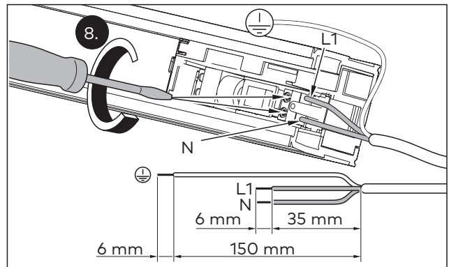
Abb. 44 Die Leitungen L1 und N anschließen
