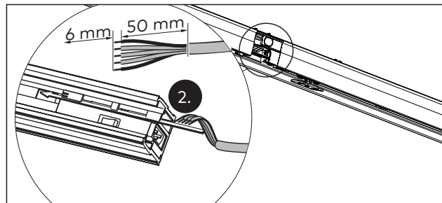
Abb. 51 Die Zuleitungen abisolieren
