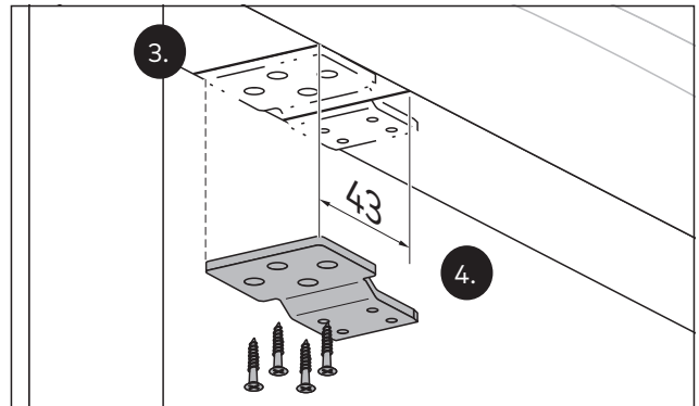
Abb. 30 Die Befestigungslasche festschrauben
