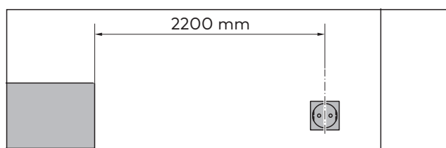
Abb. 4 Montage mit Schutzkontakt-Steckdose
