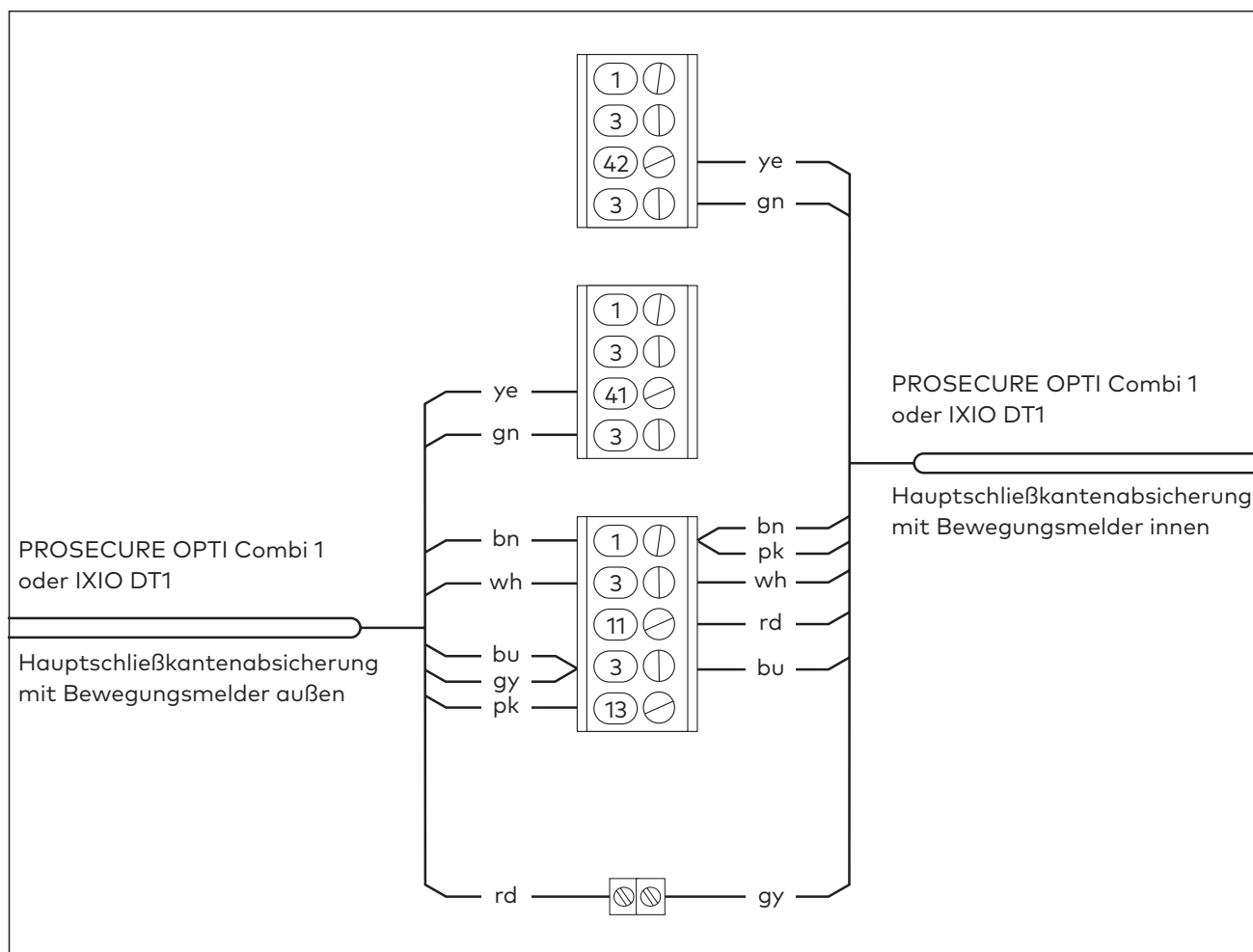
Abb. 55 Anschlussplan Schließkantenabsicherung mit Bewegungsmelder
