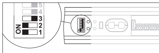
Abb. 58 DIP-Schalter
