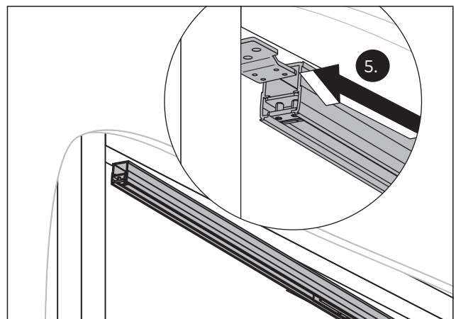
Abb. 31 Den Antrieb in die Befestigungslasche schieben
