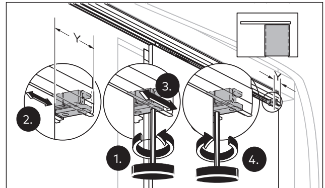
Abb. 39 Den Endanschlag auf der Anschlussseite positionieren
