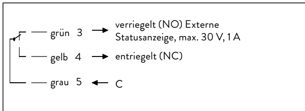
Abb. 4 Kabelfarben für das optionale Kabel-Set
