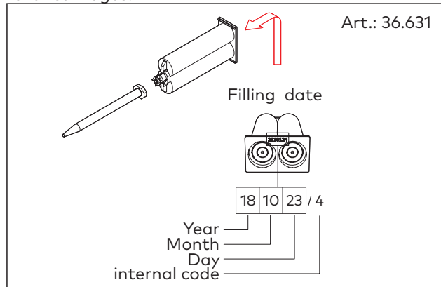
Abb. 5 Adhesive
