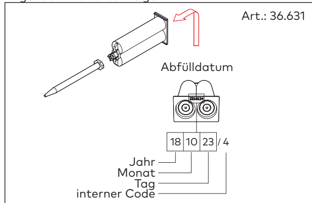
Abb. 2 Klebstoff
